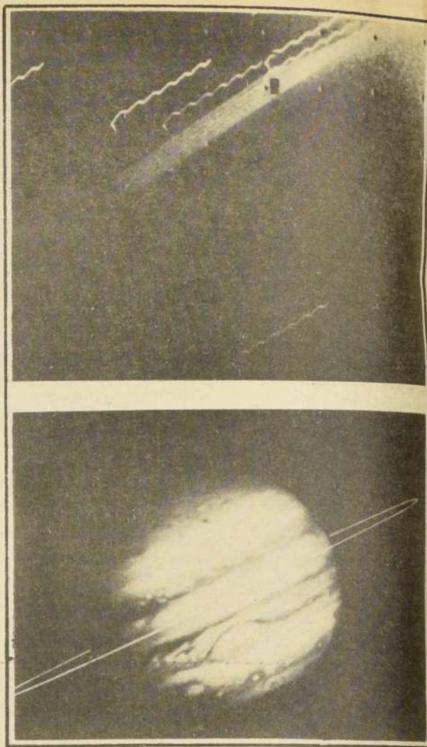
ANILLO INSOSPECHADO. — Un anillo de 30 kilómetros de espesor que rodea a Júpiter fue el descubrimiento más impactante del Voyager I. Las fotos captadas desde un millón de kilómetros del planeta.
