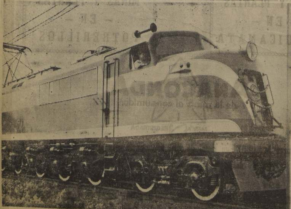
Aspecto de la locomotora de la General Electric, poderosa unidad de 210 toneladas de peso y de una potencia de 4.000 HP., que ha sido puesta en servicio entre Valparaíso y Santiago
