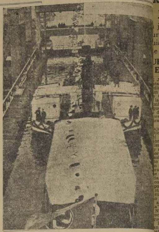
Dique de carena que es un verdadero "ascensor" para buques. En presencia del representante personal del Fuehrer, del Ministro Rudolf Hess, del almirante Raeder y otros altos funcionarios alemanes, se inauguró en Rotherhemburg el "dique de buques" alemán. El mecanismo permite levantar embarcaciones de 1.000 toneladas a una altura de 18 metros. El grabado muestra al pequeño "Hermes", entrando en el dique en Rotherhemburg.
