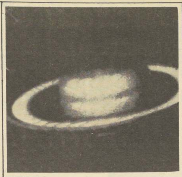
ACERCAMIENTO A SATURNO.— El hombre alcanzará una nueva frontera en su búsqueda del espacio cuando por primera vez una nave controlada desde Tierra pase cerca del Planeta Saturno y sus anillos. El Pioneer, según el programa, debe acelerar por debajo de los anillos por el flanco oscuro del planeta el sábado a las 11 A.M. (RADIOFOTO UPI UNIFAX).
