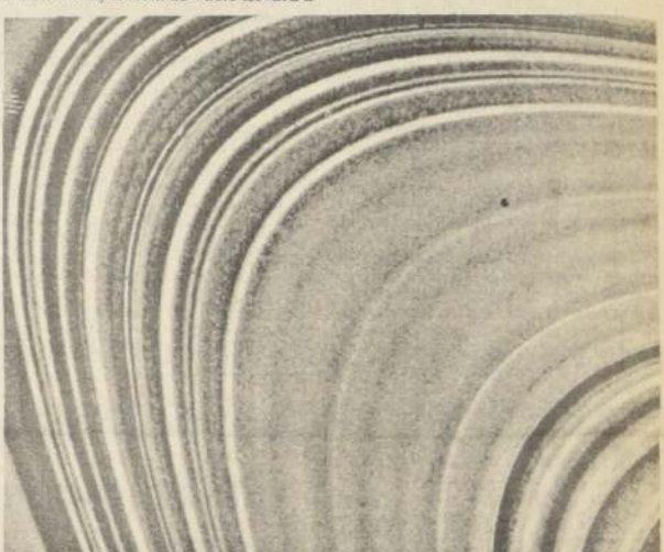
Esta vista de los anillos de Saturno se obtuvo de tres imágenes separadas tomadas a través de un filtro ultravioleta, claro y verde. Las imágenes captadas por la nave espacial Voyager 2 muestran más de 60 anillos oscuros y brillantes. Las pequeñas bandas cuadradas que se aprecian son causadas por las marcas hechas durante el proceso de revelado. En general, los anillos semi-ovalados son de un material blando y plomizo, semejante al color del hielo sucio. Las diferencias de color entre un anillo y otro se deben a los distintos componentes que conforman la compleja estructura de ellos.
