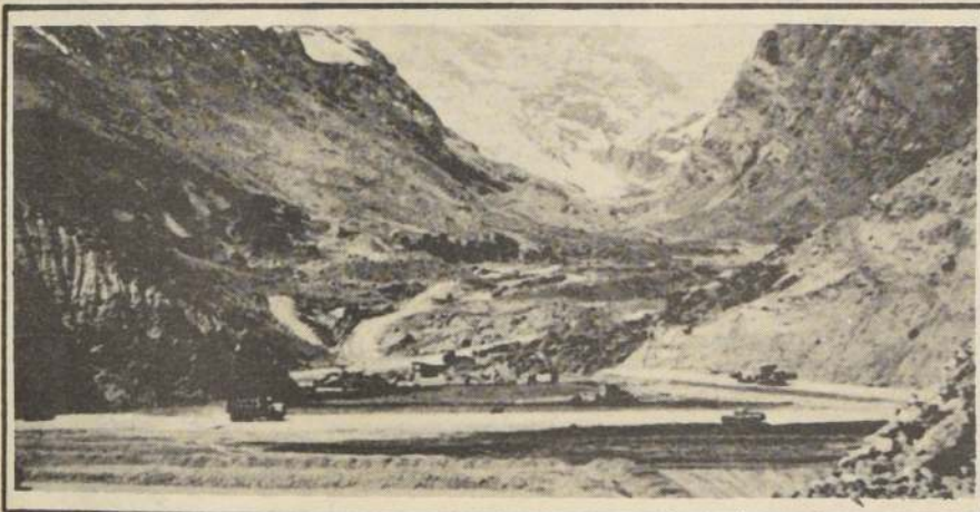
AREA DEL VALLE del río Los Leones donde se construye el nuevo embalse de relaves de CODELCO-Chile División Andina. En el grabado, la zona donde se levanta el muro que retendrá el material proveniente de la planta concentradora.
