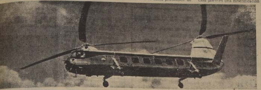
HELICOPTERO BIMOTOR BRISTOL 173, construido por la Bristol Aeroplane Company Ltd., de Bristol, Inglaterra. Puede transportar trece pasajeros, y para mantenerse en vuelo le basta uno de sus dos motores Alvis Leonides.
