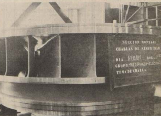
Este es sólo un repuesto de uno de los generadores Hitachi que se emplean en la Central Antuco, que operan a una velocidad de 250 revoluciones por minuto.
