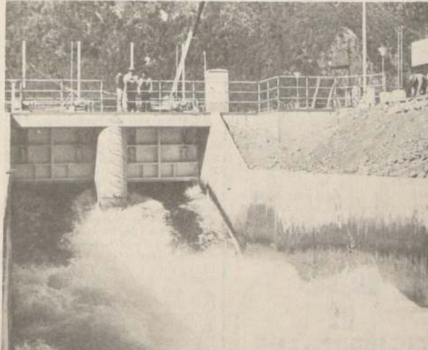
La aducción Laja que entregará su cuota de agua para el funcionamiento de la Central Antuco.
