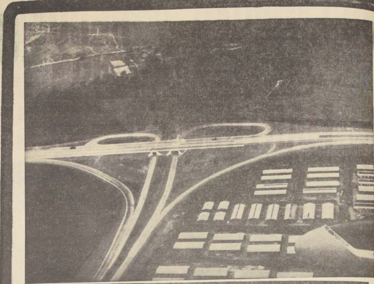
Este es el "trébol" de distribución de vías, contruido frente a Lo Espejo, en la Carretera Longitudinal Sur. El paso superior y sus pistas adyacentes permiten la rápida y segura circulación de vehículos, evitándose cualquier riesgo de accidente, especialmente choques y atropellos, tan frecuentes en los cruces carreteros. Es una de las principales obras en el tramo Santiago-Rancagua, distancia que se cubre en menos de una hora de viaje.
