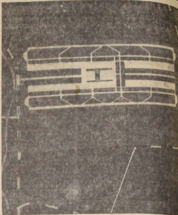
En el grabado, el plano definitivo del aeropuerto de Pudahuel destinado a convertirse en el primer campo de aterrizaje del país. Este moderno aeropuerto, cuyas obras están experimentando efectivo progreso, se está levantando al lado norte del río Mapocho, a unos 2.200 metros sobre el nivel del mar y tiene una pista de 3.200 metros.
