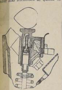
Como funciona el levanta-válvulas hidráulico
