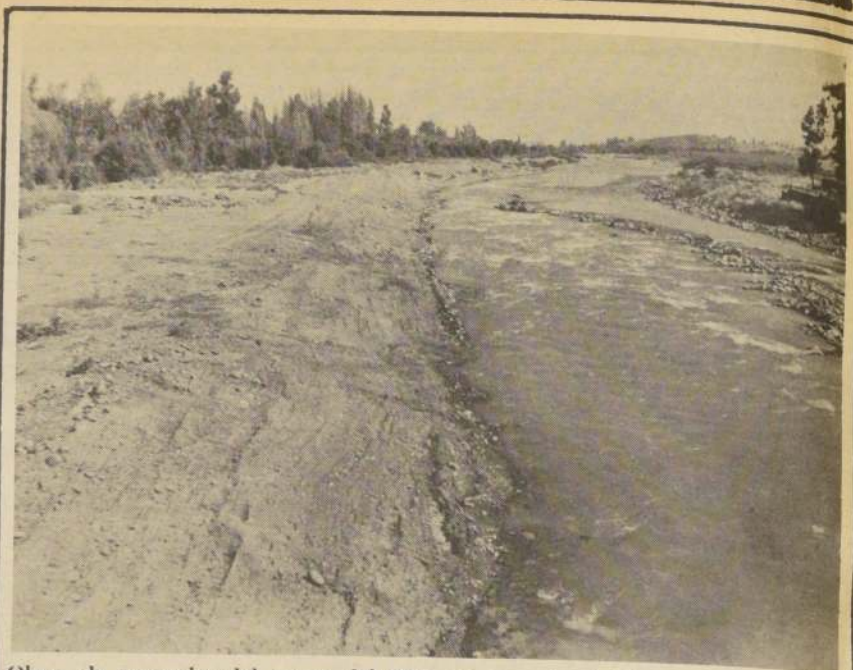
Obras de ensanche del cauce del Río Aconcagua y de defensa de sus riberas en el sector del Puente García, en Los Andes.
