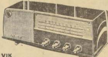
VIK Receptor de sobremesa. Onda larga y dos ondas cortas. 8 transistores. Funciona con solo 4 pilas de 1,5 volts. Enchufe de audifono. E° 12 AL MES
