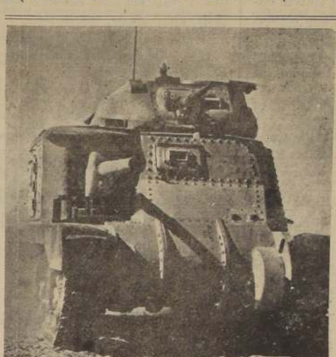
Los nuevos tanques norteamericanos "General Grant" han sido usados en la nueva ofensiva aliada en el frente del desierto. Arriba: un tanque con un cañón de 37 mm. y con otro de 75 mm., y poderosamente blindados, han hecho estragos entre las divisiones panzer del enemigo.
