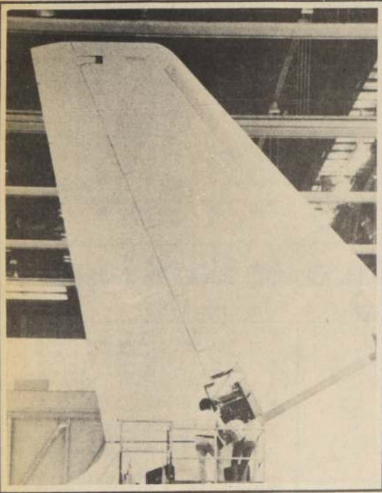
MENEANDO LA COLA. — Los técnicos de la Lockheed-California se ven diminutos junto a la enorme cola de un TriStar L-1011. Están realizando ajustes en el mecanismo hidráulico del timón del aparato en la planta de la compañía en Palmdale. El timón, de ocho metros de alto y 385 kilos de peso, gira a la izquierda o derecha para cambiar la dirección del vuelo. (CPS).
