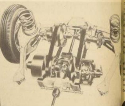
EL PEQUEÑO GIGANTE. El Mini Cooper, es el tipo de coche que rueda en calles y pistas latinoamericanas. De un perfecto equilibrio, fabricación es un derecho de imaginación y de cálculo útil. Aquí, esquematizados, sus sistemas de suspensión y transmisión.
