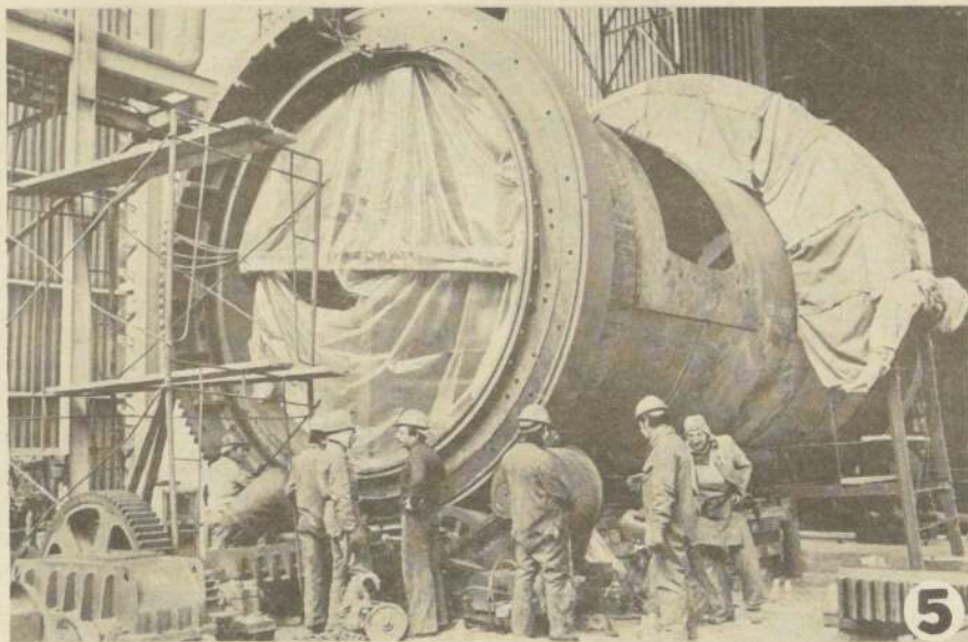
5 HORNO BASCULANTE para refinado a fuego, cuya construcción ya se terminó.
