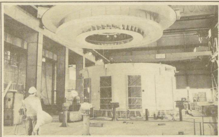
La ENDESA construye en Ñuble la nueva central Antuco, que generará 300 mil kilowatts-hora. Reforzará la energía eléctrica que circula desde Atacama hasta Chiloé. Trabajan en esta obra 2.600 personas.
