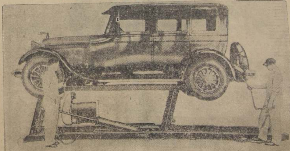
La plataforma levanta el automóvil hasta la altura que más convenga para proceder a la lubricación del coche.
