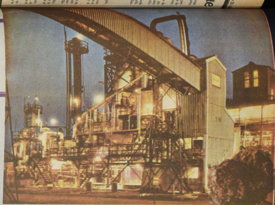
Una planta carboquímica para producir bencina de carbón.
