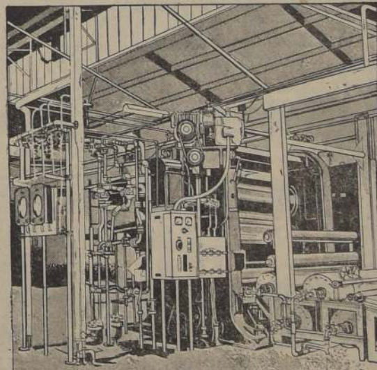
Aspecto parcial de la Calandria gigante, empleada en uno de los procesos de elaboración de Plásticos Flexibles. Es la única de este tipo montada en Sud-América.
