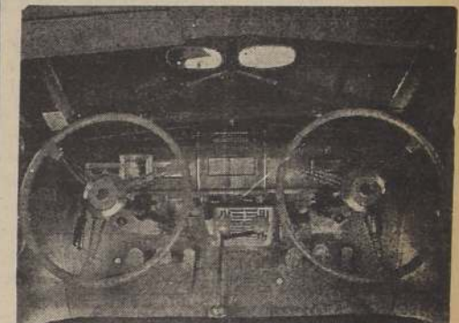
Vista interior del coche Studebaker con mandos gemelos. Nótese los volantes de dirección, pedales de frenos, de embrague y de acelerador dobles; dos palancas de freno de mano, dos arranques y dos espejos retrovisivos. La palanca de cambio de velocidades está ahorquillada, lo que permite al instructor guiar al aprendiz en el cambio correcto de los engranajes.
