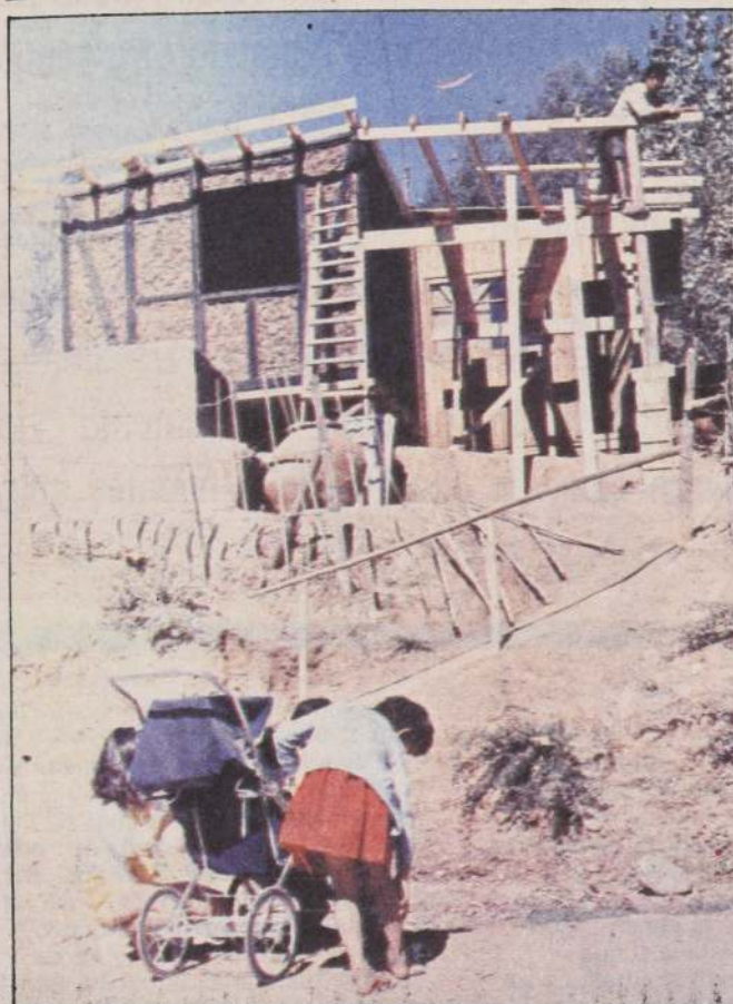
El antiguo adobe de las casas y los tejados de greda no resistieron los bruscos movimientos de la tierra en Melipilla (arriba). En la siguiente foto se muestra una nueva técnica de construcción para Pomaire. Se trata de la tabiquería de adobe que otorga mayor resistencia a la edificación.
