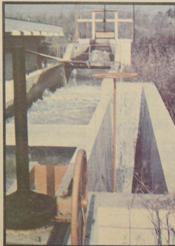
A gran velocidad, las aguas son sometidas al tratamiento denominado "mezcla rápida", en una primera etapa.
