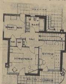
Segundo piso
