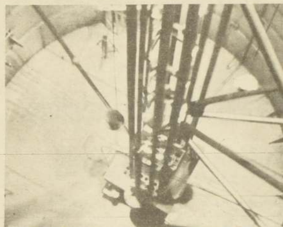
Piscina del reactor en cuyo fondo está sumergido un trozo de uranio 235. Las barras verticales son para controlar el proceso.
