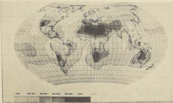
Mapa indicativo de la intensidad de la radiación solar. En diversas partes del mundo, incluso en Chile, se está recurriendo, en forma experimental, a la energía solar para desalinizar el agua de mar.
