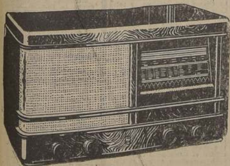
Modelo 312: Superheterodino de extraordinario rendimiento en onda corta. Equipado, además, con el famoso triodo-hexodo para estabilizar la frecuencia.
