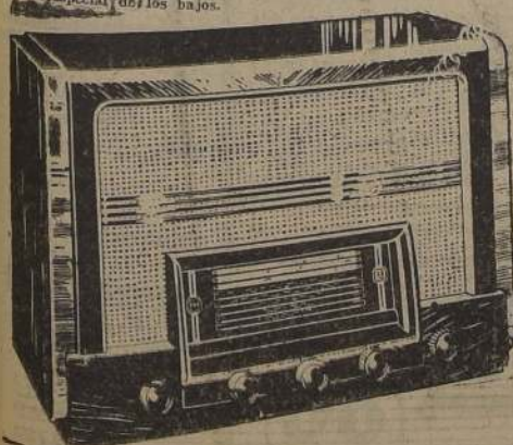
Modelo 316: Superheterodino de tubo con sintonización de bandspread calibrado. Sintonizador de permeabilidad y dial calibrado en bandas de 13, 16, 20, 25 y 30 metros. Amplificación especial de los bajos.
