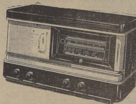
Modelo 314: Superheterodino equipado con corrección automática de calidad, nuevo circuito de contrarreactión para la pureza del tono. Condensador de sintonización termostático.
