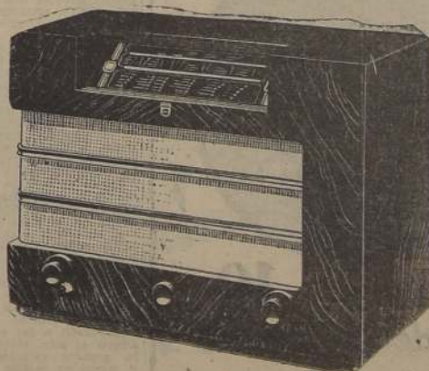
Modelo 232-V: Superheterodino de batería, equipado con válvulas para corriente de red, alimentado completamente por un acumulador de 6 volts, en combinación con un vibrador Philips.
