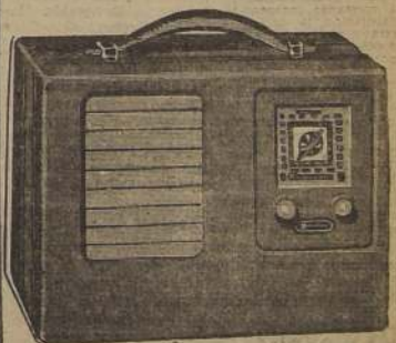
C. J. 263: Radio portátil de batería Superheterodino de 5 tubos de onda larga, con antena interior. De gran alcance y selectividad. Elegante gabinete-maleta de color beige
