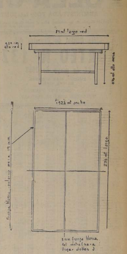
PLANO CON LAS MEDIDAS REGLAMENTARIAS DE UNA MESA DE TENIS DE MESA. ESCALA 1:20.
