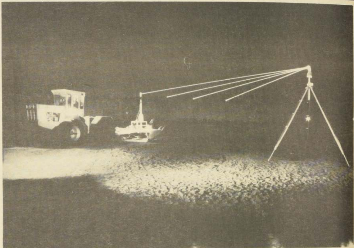
Tractor guiado con Laser. — La función de estos tractores removedores de tierra, guiados por rayos laser, que se emplean en el laboratorio de Conservación de agua de Phoenix, Arizona, es la de permitir una mayor precisión en aplicar la cantidad exacta de agua de regadío necesaria —en forma igual y rápida.— Las cuatro exposiciones de esta fotografía muestran la luz enviada a una escarbadora movida por un tractor. El receptor intercepta el laser y mantiene la posición de las cuchillas de la escarbadora en la adecuada elevación de terreno.
