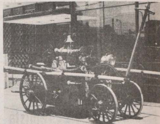
En la tercera Compañía del Cuerpo de Bomberos de Santiago se encuentra esta bomba a palanca fabricada en Boston el año 1864 y puesta en servicio en septiembre de ese mismo año. Una de las particularidades de esta reliquia es que aún funciona en perfectas condiciones.
