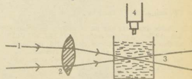
Esquema del ultramicroscopio en que se demuestra el efecto Tyndall
