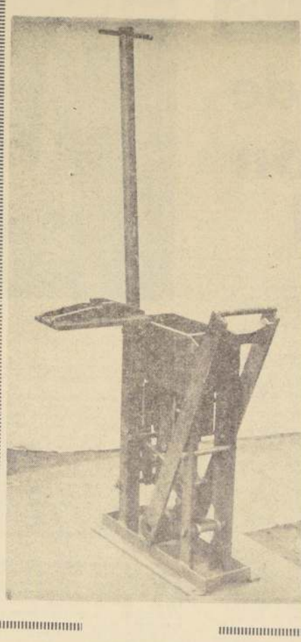
Ochocientos bloques suelo cemento puede fabricar diariamente esta máquina, que fue inventada por el técnico del Servicio de Cooperación Técnica, Juan Pacheco. La máquina permitirá disminuir apreciablemente los costos de autoconstrucción.
