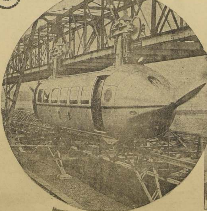
Esta vista del railplano muestra cómo el vehículo está suspendido de los rielles. Nada descansa en la estructura situada debajo de él, la cual solamente existe para el contrabalanceo del aparato.
