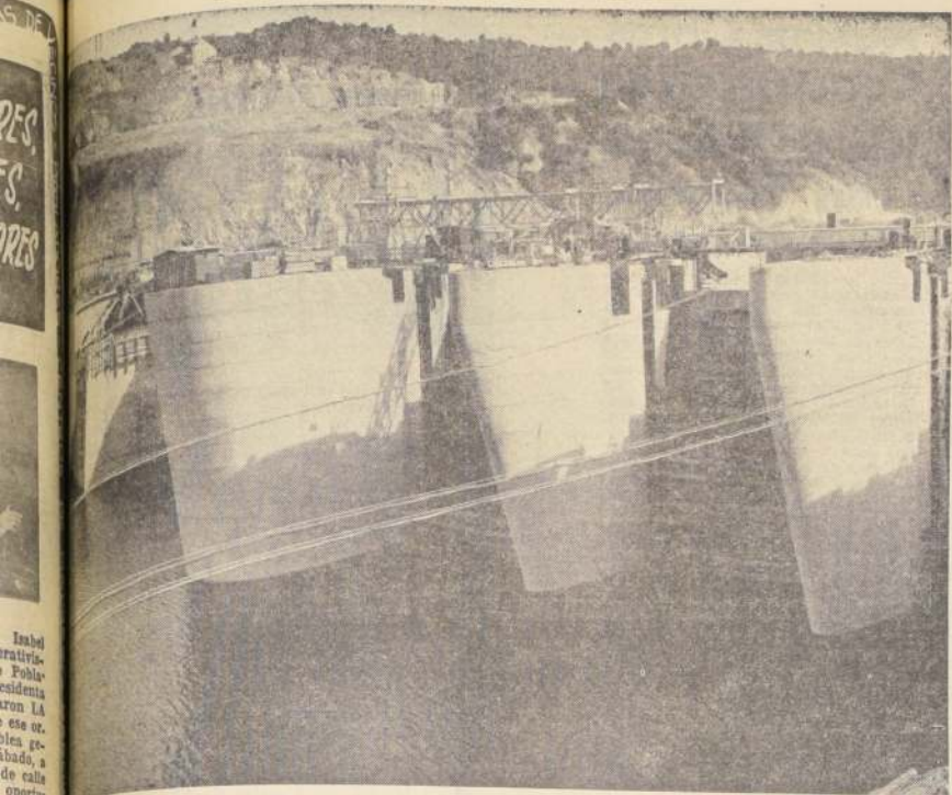
La Central Hidroeléctrica de Rapel, un coloso de la ingeniería chilena. Esta se encuentra ubicada en Quelantaro, a 45 kilómetros del río Rapel, y cuenta con generadores, dos de los cuales ya están en funcionamiento, con capacidad de 70 mil kilowatts cada uno. El costo total de la obra asciende a cien millones de dólares. El muro de contención que se inició en el mes de mayo y posee 111 metros de alto, constituyéndose en el primero de su especie en el país y uno de los cuatro mayores de América Latina.
