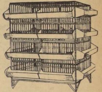
Batería de recría, tipo Buckeye, para 400 pollos hasta las doce semanas
