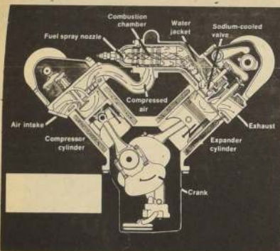
Diagrama del nuevo motor Warren, limpio y económico en su uso
