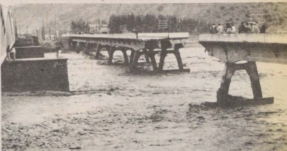
Personal de Vialidad y del Comando de Ingenieros del Ejército instala un puente mecánico para restablecer el tránsito en el Camino Longitudinal Sur, mientras se supera la emergencia.
