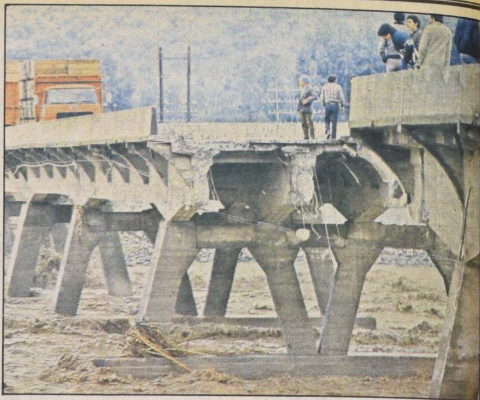
Viaducto cortado sobre el río Tinguiririca, hasta donde se envió un puente mecánico, tipo Bailey, para restablecer el tránsito vehicular en las próximas horas.
