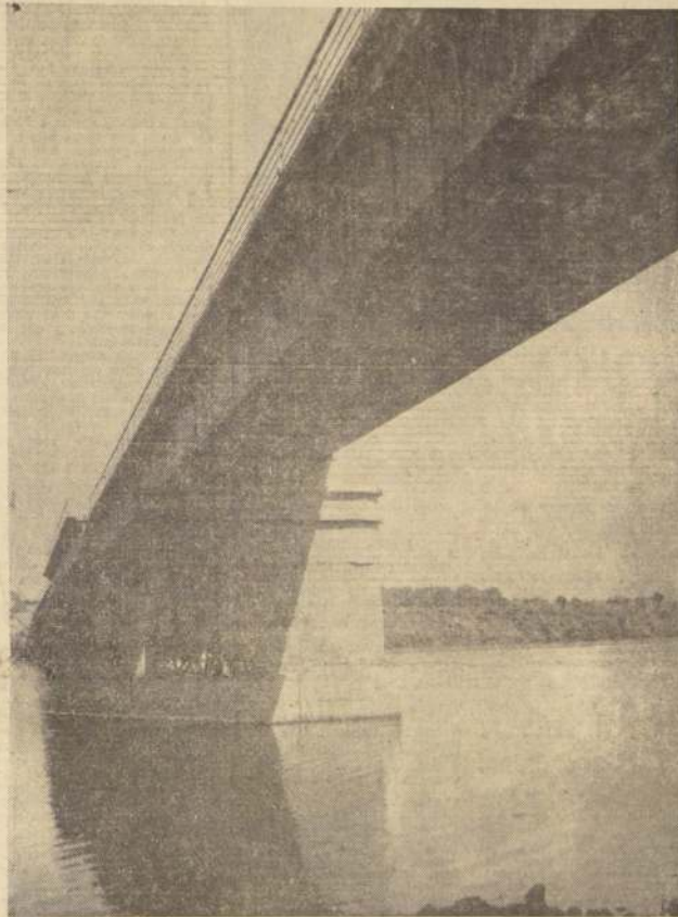
Desde hoy 36 mil nuevas hectáreas regadas se incorporan a la producción agropecuaria de la Zona Central, al entregarse las obras de regadío en las provincias de Linares y Talca. En el grabado, el puente sifón construido sobre el río Loncomilla, en concreto pretensado de 2.400 metros de largo, y el agua se escurre entre las vigas internas, en cantidad de 6,3 metros por segundo.
