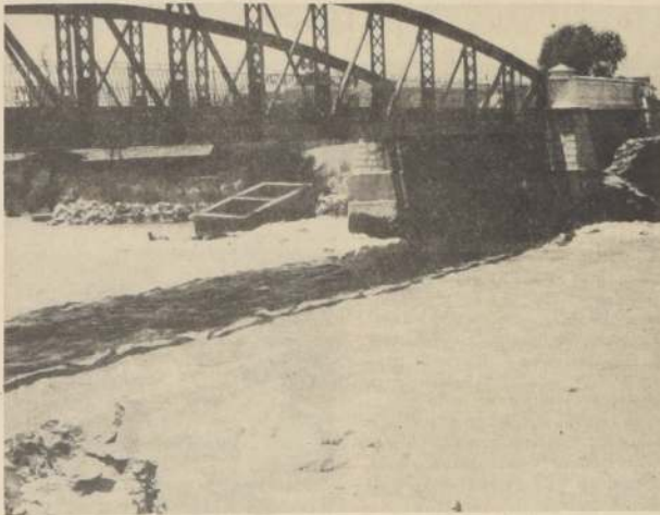
El antiguo puente de acceso a San Felipe, con más de un siglo de uso, será reemplazado por una moderna construcción. Se observa una de las primeras fundaciones que fueron arrastradas por el gran caudal del río Aconcagua.
