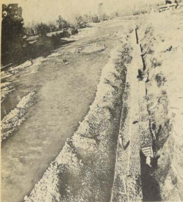
A las defensas de enrocados en el río Mapocho se sumaron los modernos "gaviones", sistema internacional de gran efectividad que se seguirá utilizando en Chile en puentes y caminos de crecidas fluviales.
