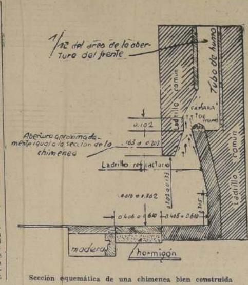
Sección esquemática de una chimenea bien construida.
