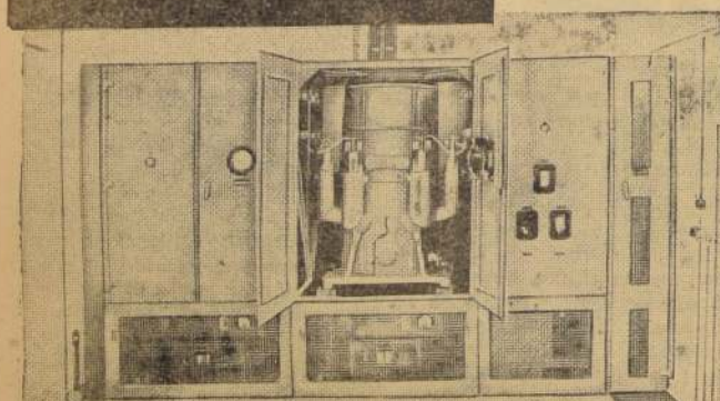
Uno de los 20 equipos rectificadores al arco de mercurio, sin bomba, enfriado por aire, fabricado por English Electric para los Ferrocarriles de Holanda.
