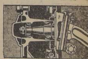
NUEVOS MUNONES MAS GRANDES—Un factor aumentado de seguridad para los camiones de 340 cms. y 399 cms. Los ejes nuevos más grandes en partes de mayor tamaño. La superioridad más grande de los ejes y de los ejes reduce el desgaste. El nuevo diseño del eje mejora la acción de frenado.
