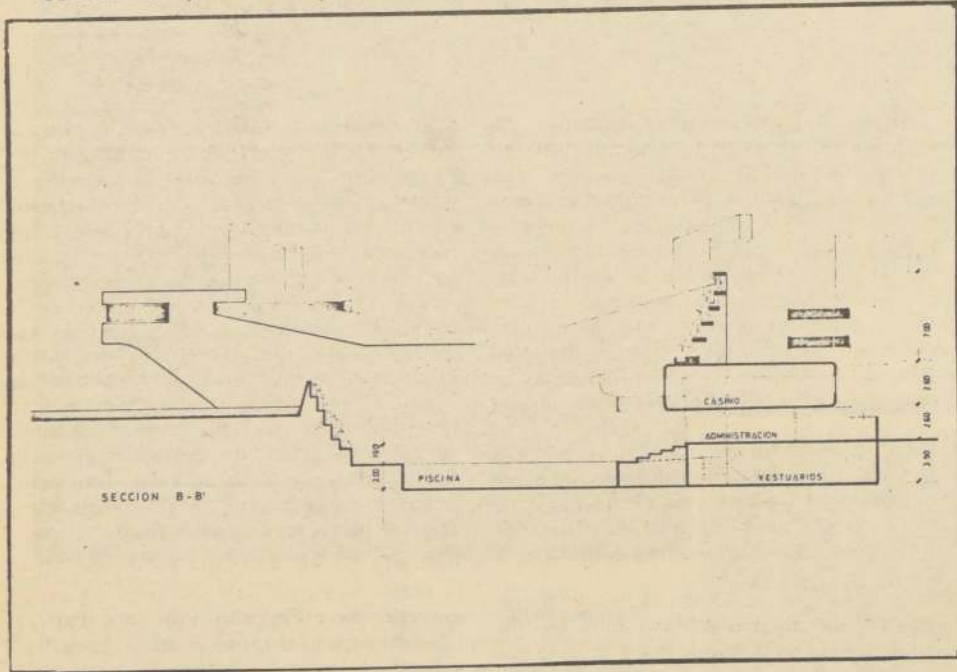
La sección muestra la estructura del edificio y los distintos niveles del techo corredizo.
