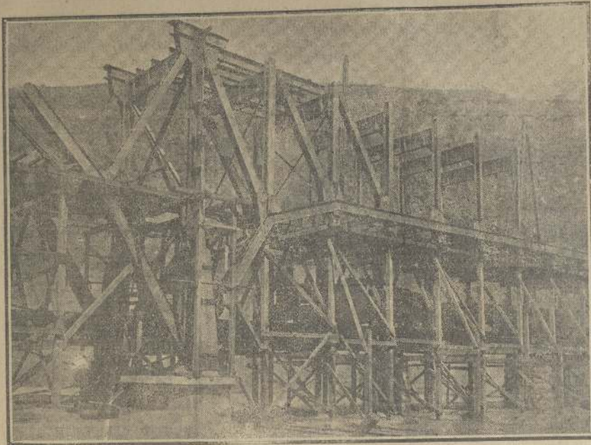
Estado actual del puente «Las Cucharas», entre Salto y Quilpué, de la doble vía.
