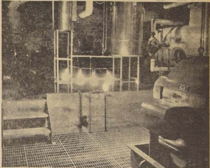
Se tratan una fotografía de la primera planta de energía atómica instalada en los Estados Unidos de Norteamérica. Cuatro ampolletas de luz eléctrica permanecen encendidas para demostrar el primer empleo que se conoce hasta ahora de una planta eléctrica movida por energía nuclear. Las ampolletas han sido encendidas por la electricidad emanada de un generador que está a la derecha, el que se mueve a su vez por el calor que emite un reactor, alimentador experimental recientemente construido. (Foto UNITED PRESS-ACME.)
