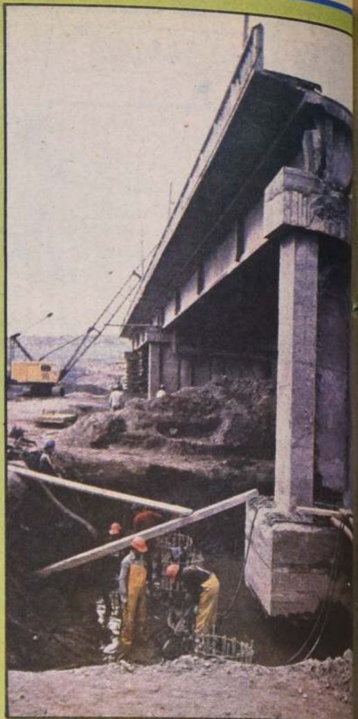
El Departamento de Puentes del Ministerio de Obras Públicas construye las dos últimas cejas que permiten la habilitación definitiva del puente Lo Gallardo, que será entregado al uso el próximo 10 de diciembre.
