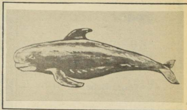
EJEMPLAR de calderón negro o "ballena piloto" cuya muerte masiva preocupa a los ecólogos.
