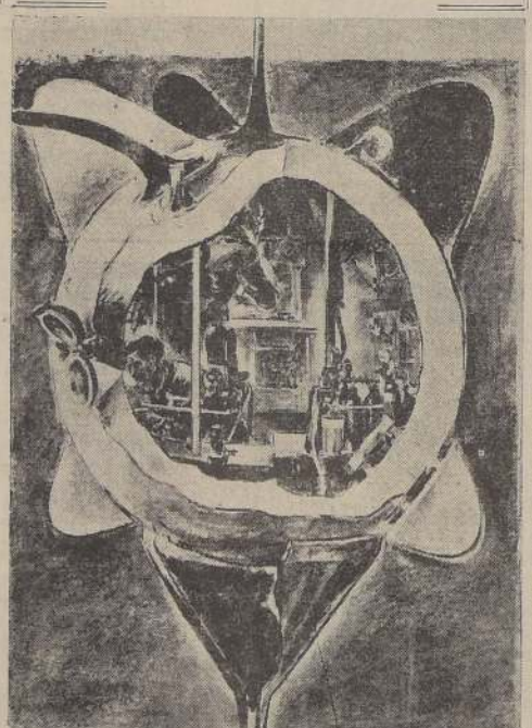
A una profundidad de 10.000 metros, la presión alcanza a 1.000 atmósferas de presión. La original esfera ideada por el profesor Piccard será construida con electón, aleación capaz de soportar dicha presión. Las 8 aletas de la esfera están destinadas a mantener la verticalidad del descenso a las profundidades.
